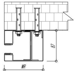
RAY DẪN HƯỚNG GUIDE RAILS
