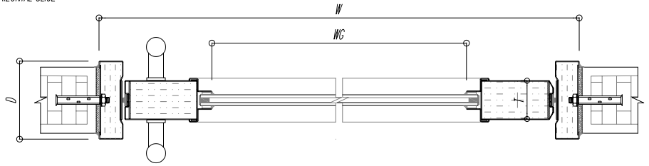
MẶT CẮT NGANG CỬA ĐƠN SINGLE LEAF HORIZONTAL SLICE
