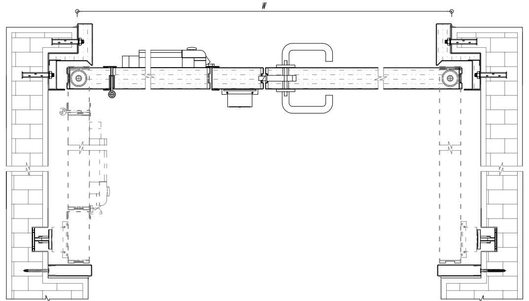
MẶT CẮT NGANG CỬA ĐÔI - 90° DOUBLE LEAF HORIZONTAL SLICE - 90°
