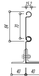
NAN CỬA SLAT
