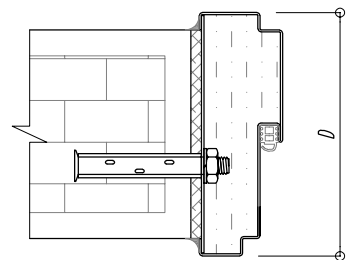
CỬA KHÔNG PHẠO CASELESS
