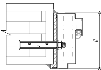
CỬA MỞ RA NGOÀI PHẠO PHÍA NGOÀI OUTWARD-OPENING/OUTER-CASING
