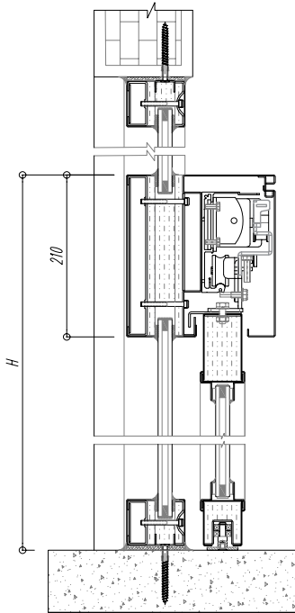
MẶT CẮT ĐỒNG VERTICAL SLICE
