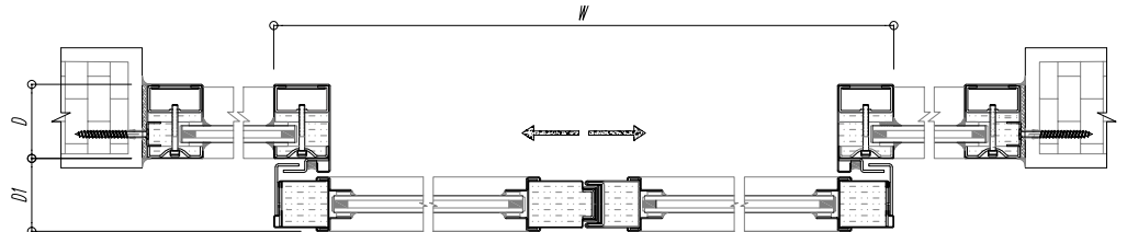
MẶT CẮT NGANG CỬA ĐÔI DOUBLE LEAF HORIZONTAL SLICE
