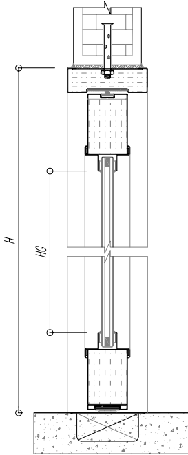
MẶT CẮT ĐỨNG VERTICAL SLICE
