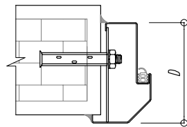
CỬA MỞ TRONG PHẠO PHÍA NGOÀI INWARD-OPENING/OUTER-CASING
