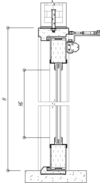
MẶT CẮT ĐỨNG VERTICAL SLICE
