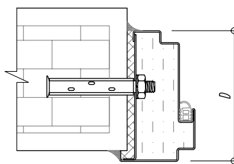
CỬA MỞ VÀO TRONG PHẠO PHÍA NGOÀI INWARD-OPENING/OUTER-CASING
