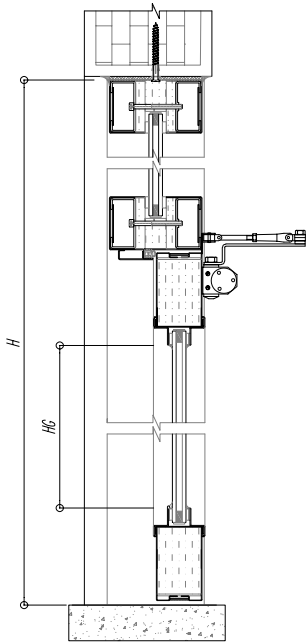
MẶT CẮT ĐẲNG VERTICAL SLICE
