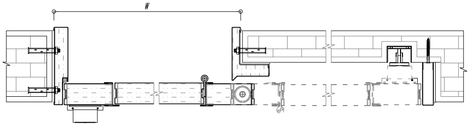
MẶT CẮT NGANG CỬA ĐÔI - 90° DOUBLE LEAF HORIZONTAL SLICE - 90°
