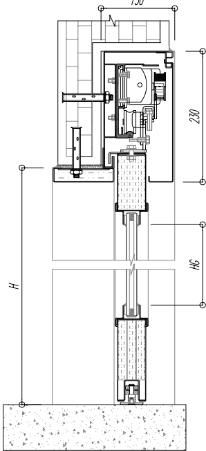
MẶT CẮT ĐỨNG VERTICAL SLICE
