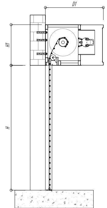
RAY DẪN HƯỚNG GUIDE RAILS
