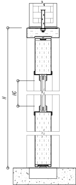
MẶT CẮT ĐỨNG VERTICAL SLICE
