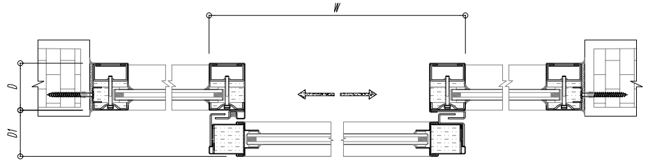
MẶT CẮT NGANG CỬA ĐƠN SINGLE LEAF HORIZONTAL SLICE
