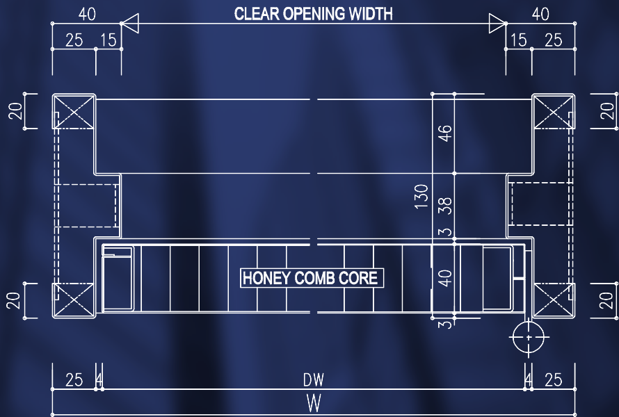
MẶT CẮT NGANG/ Horizontal section
