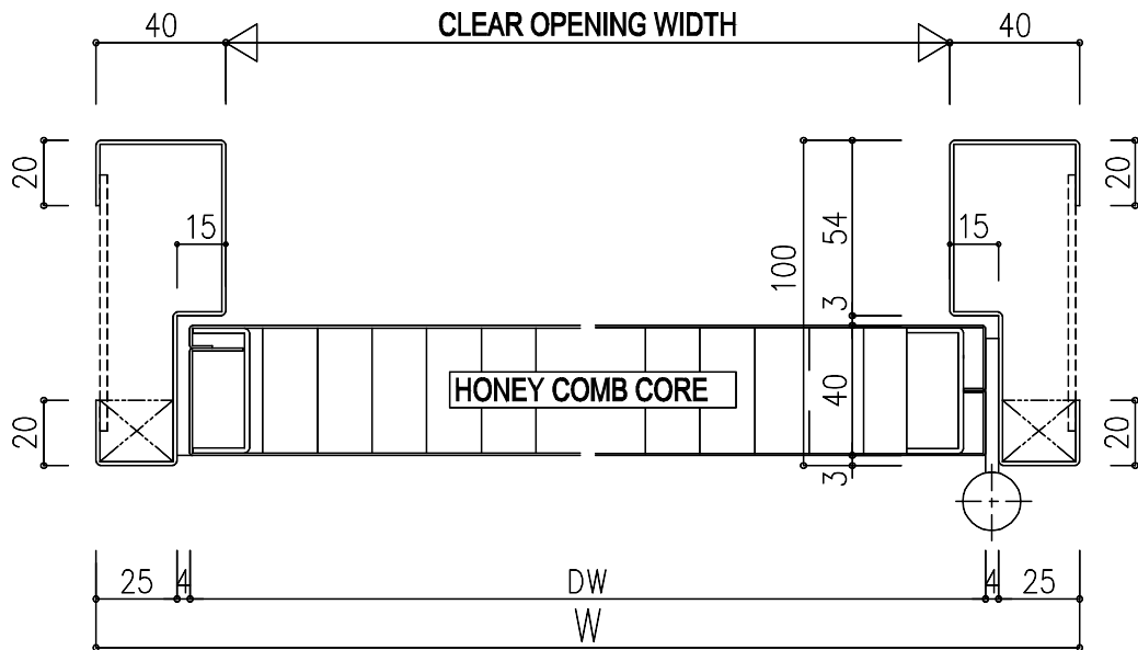
MẶT CẮT NGANG/ Horizontal section
